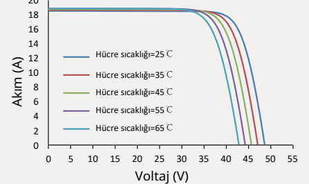
Akım-Voltaj (615W)
