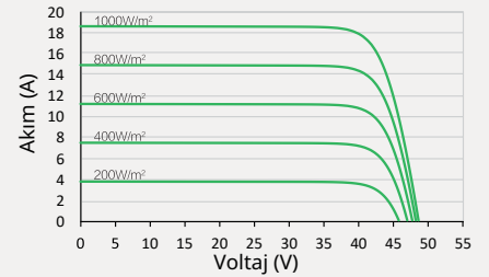
Güç-Voltaj (615W)
